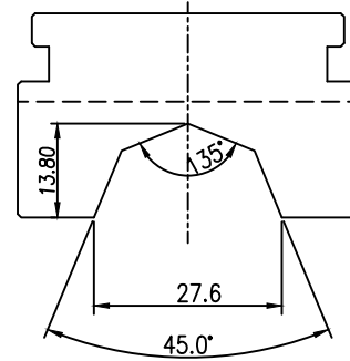
lower die 下模
