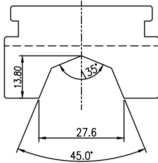
upper die 上模
